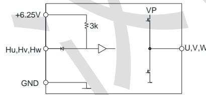
接口电路
